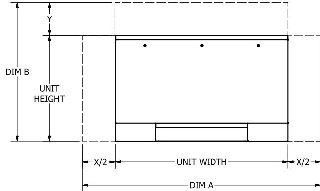
Model VFE Parametric Increments
